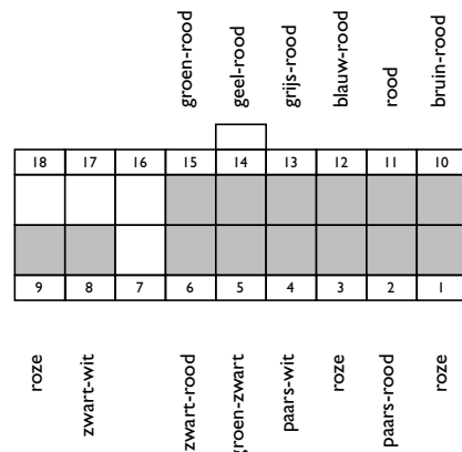
Achterzijde 18 polige connector
