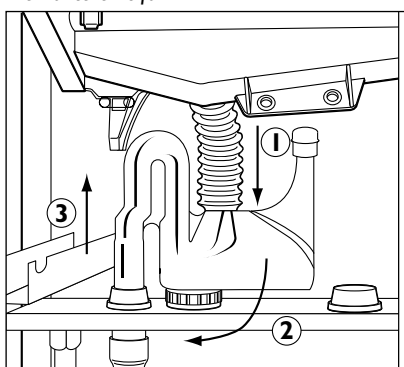
Figuur 3.2.4 Demonteren sifon
