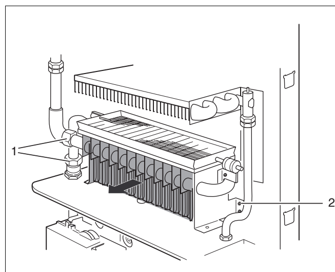
Afb. 42 Brander eruit nemen
