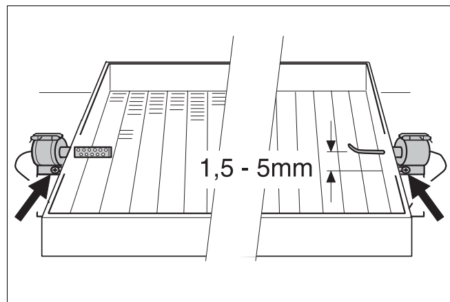
Afb. 41 Gloeiplug en ionisatiepen
