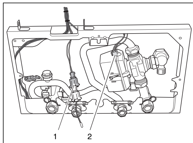
Afb. 14 Aansluiting boilersensor bij externe boiler
