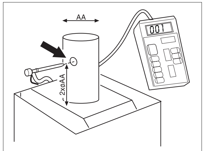
Afb. 34 Meetplaats op de rookgasafvoerleiding
