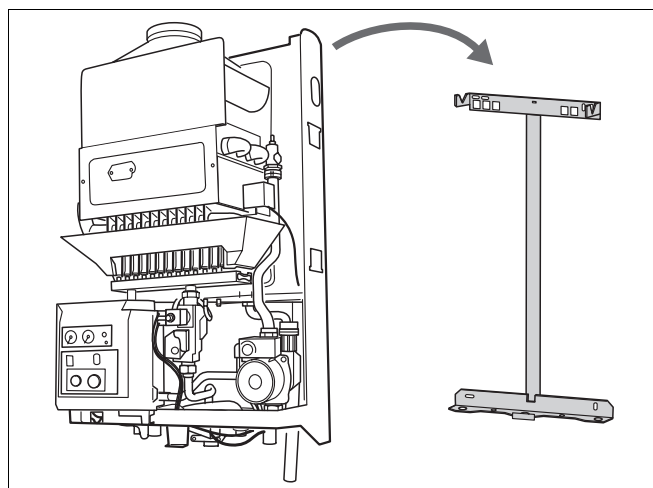
Afb. 11 Montage
