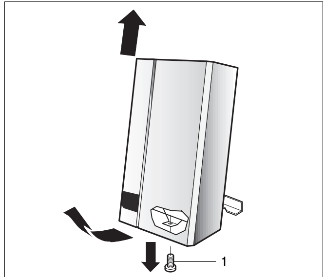
Afb. 38 Mantel aanbrengen
