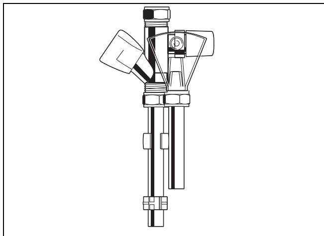
Afb. 8 KIWA gekeurde inlaatcombinatie
