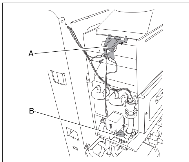
Afb. 35 Losschroeven van de sensor
