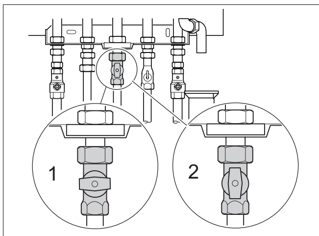
Afb. 23 Gaskraan
