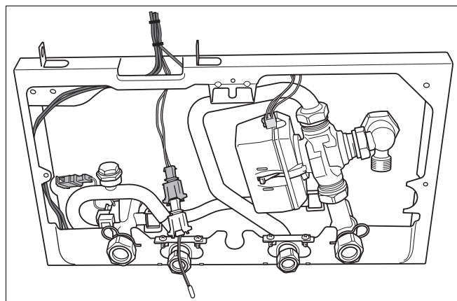
Afb. 27 Warmwatervoeler
