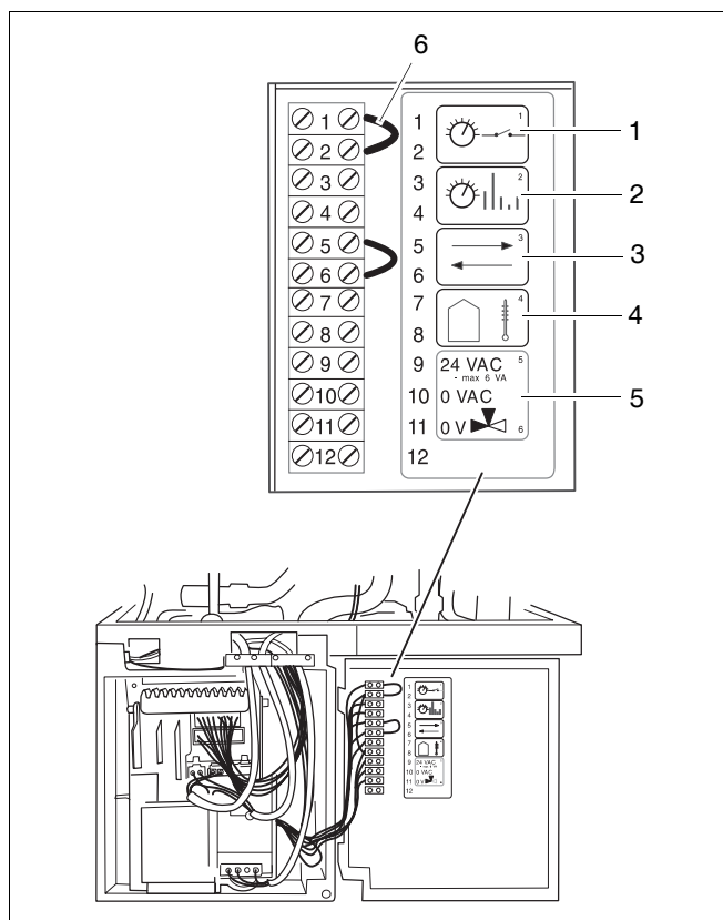
Afb. 13 Aansluiting thermostaat
