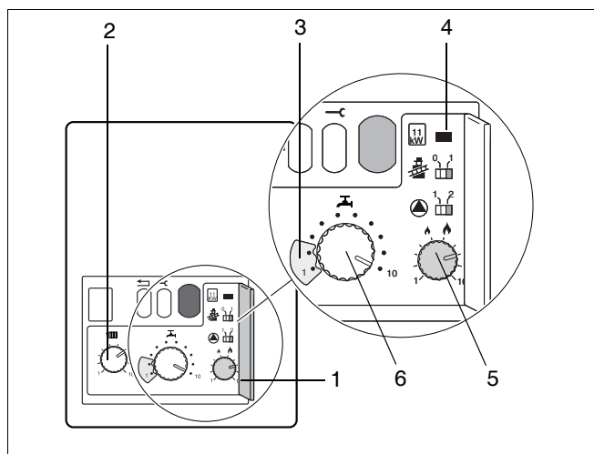
Afb. 25 Bedieningsniveau
