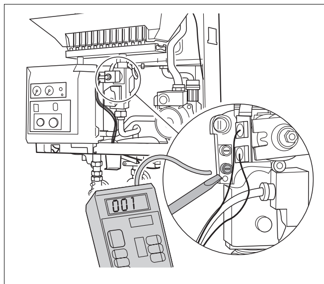
Afb. 30 Gasvoordruk meten
