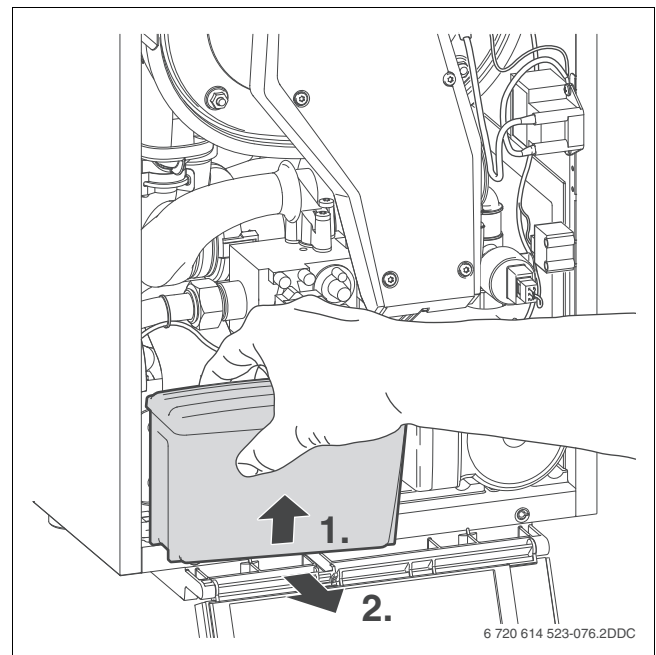
Afb. 30 Verwijderen branderautomaat
