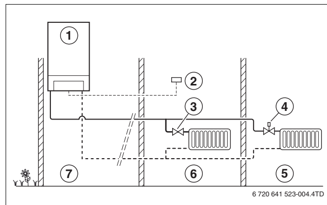
Afb. 17 Regelprincipe ruimteregeling
