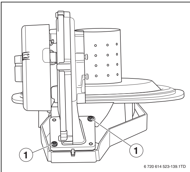
Afb. 49 Demonderen ventilator
