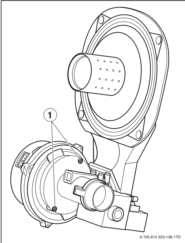
Afb. 48 Demonderen venturi
