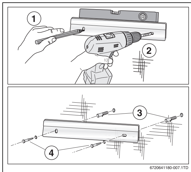
Afb. 13 Ophangbeugel monteren
