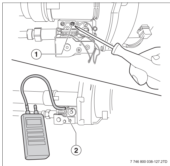
Afb. 68 Gas-luchtverhouding controleren
