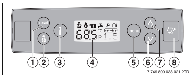
Afb. 67 Bedieningspaneel
