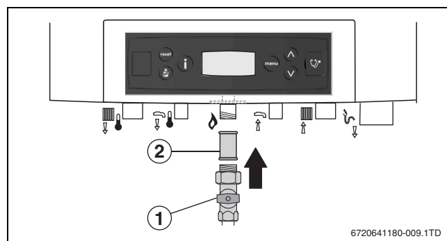
Afb. 15 Aansluiting gaszijdig
