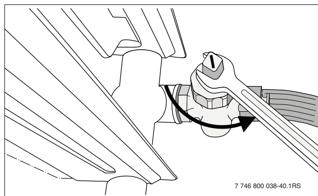
Afb. 46 Aftappen van de cv-installatie
