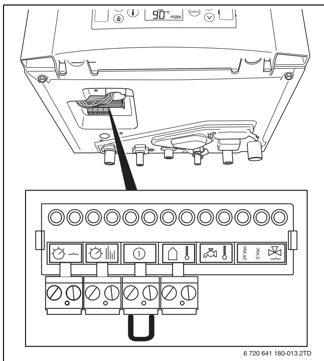
Afb. 21 Locatie aansluitstrook
