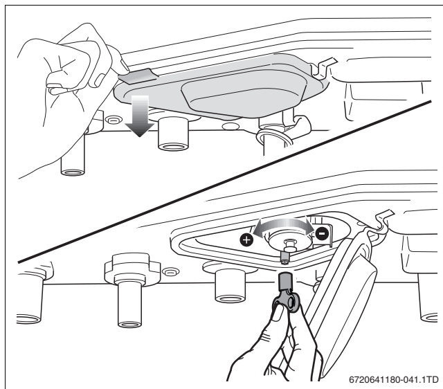
Afb. 74 Instellen uitstroomhoeveelheid tapwater
