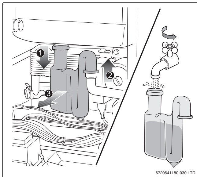
Afb. 33 Sifon uitnemen en vullen
