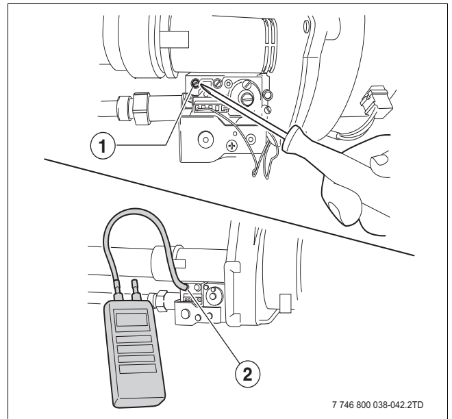
Afb. 65 Gasvoordruk meten
