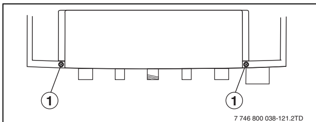
Afb. 31 Bedieningspaneel demonteren
