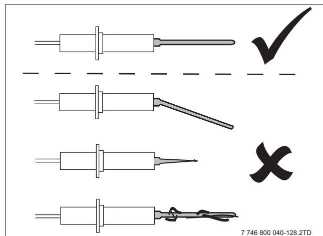
Afb. 57 Ionisatie-elektrode inspecteren
