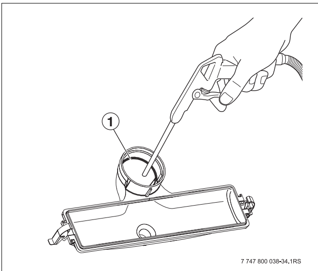
Afb. 64 Condensbak reinigen
