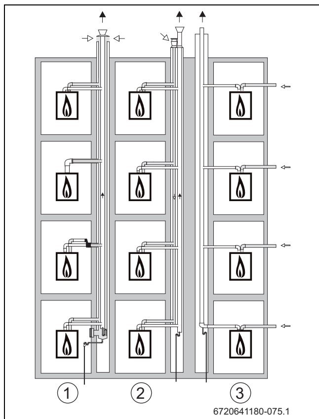
Afb. 20 CLV-systemen
