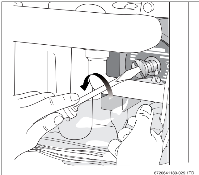
Afb. 32 Ontluchten cv-pomp
