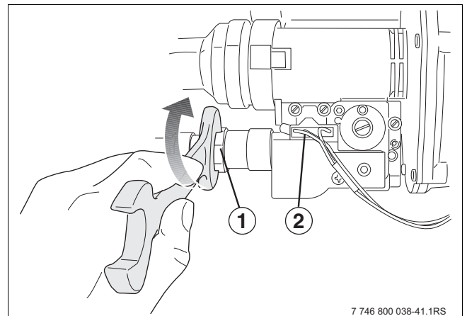
Afb. 49 Aansluitingen op het gasregelblok loshalen
