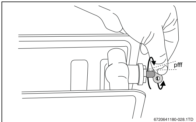
Afb. 30 Ontluchten verwarmingslichamen
