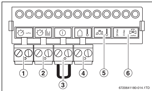
Afb. 22 Aansluitstrook
