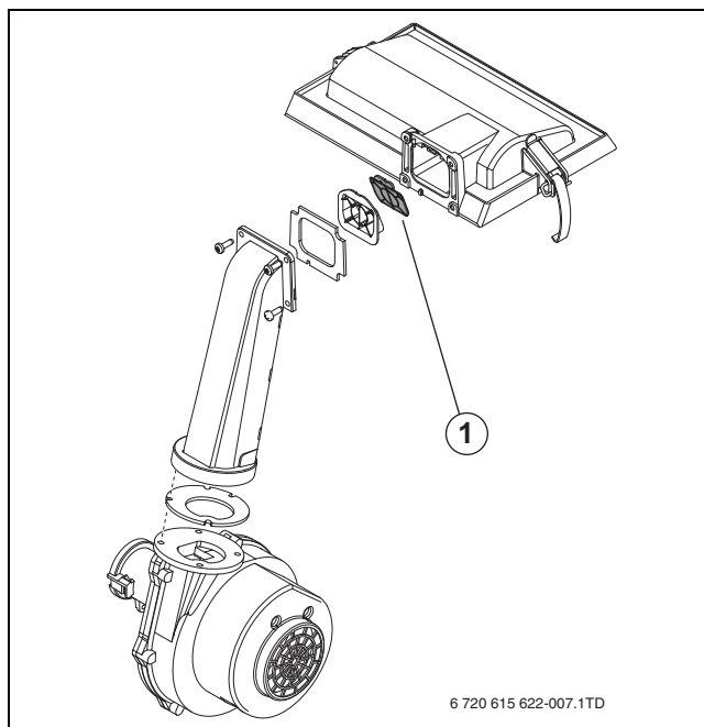
Afb. 54 Terugslagklep
