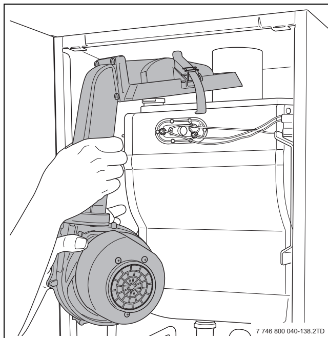
Afb. 53 Branderdeksel met gas-luchteenheid verwijderen
