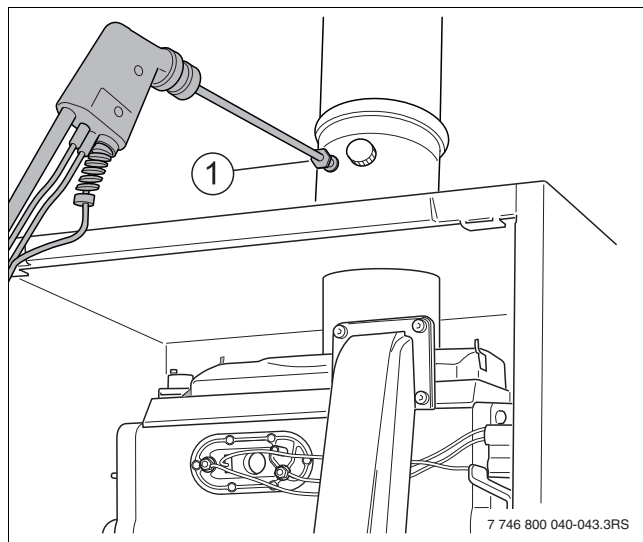
Afb. 72 Koolmonoxidegehalte meten
