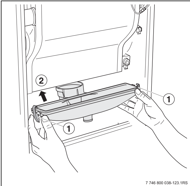
Afb. 63 Condensbak verwijderen
