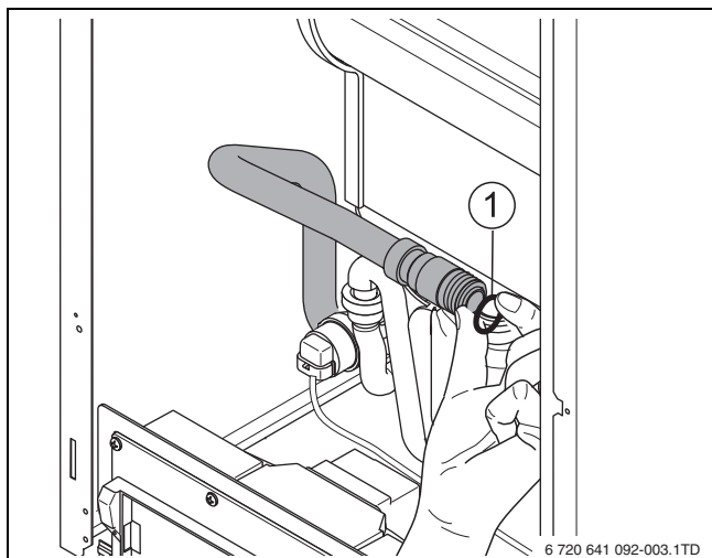
Afb. 60 Vlakke afdichtring gasleiding vervangen
