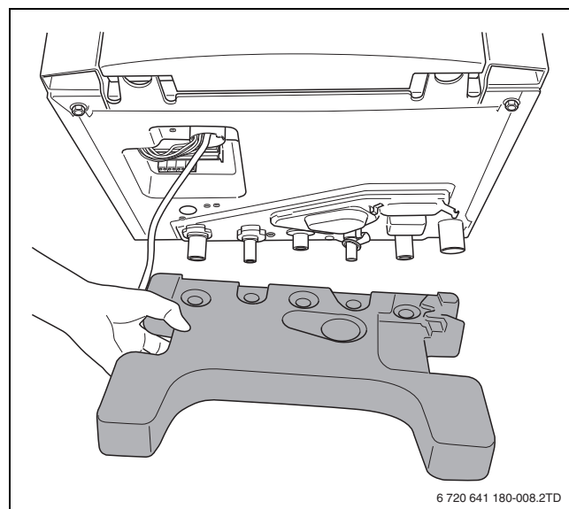
Afb. 14 Verwijderen beschermkap (zwart)
