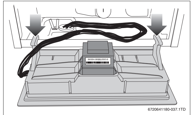
Afb. 48 Bedieningspaneel ophangen
