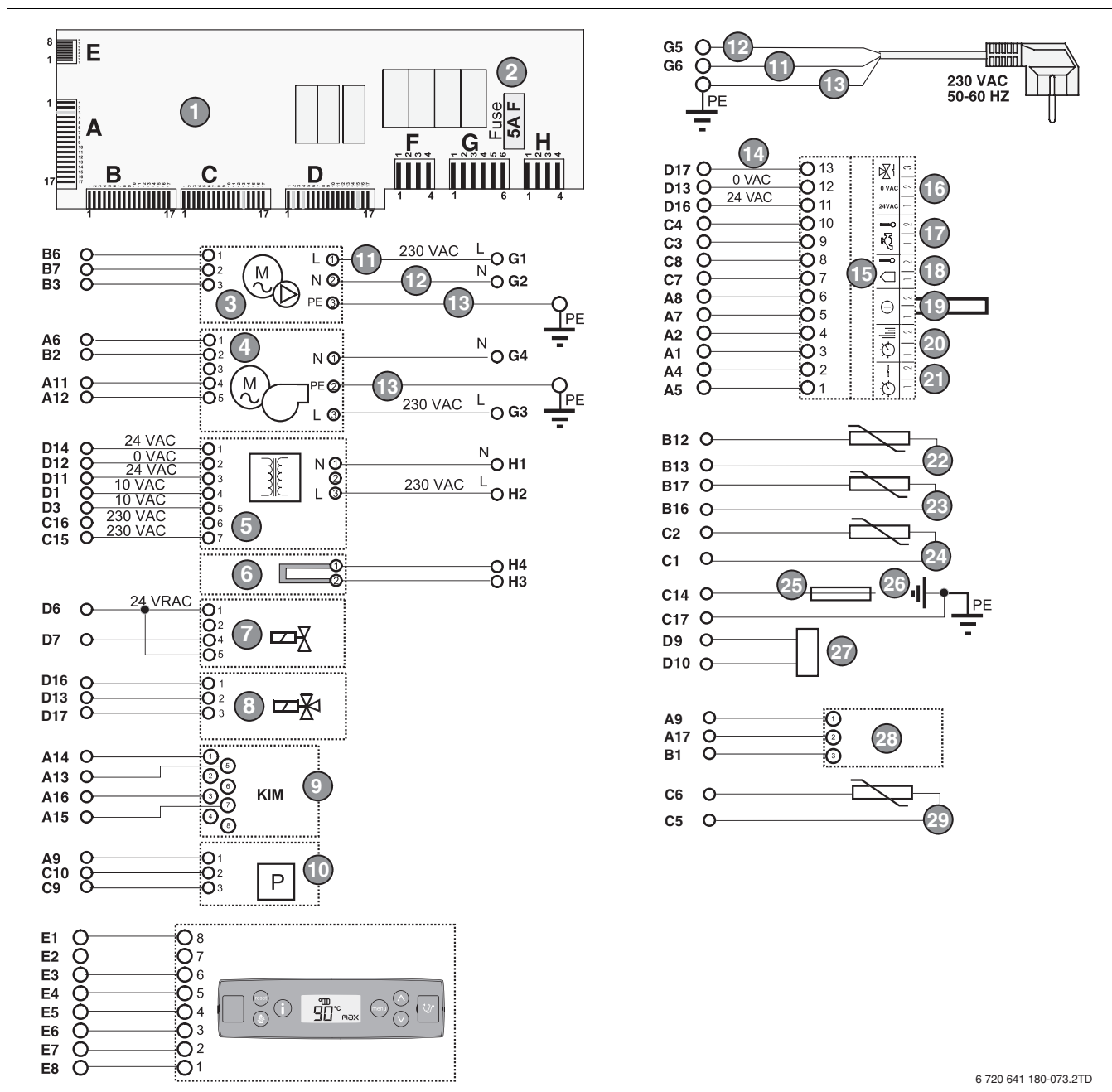
Afb. 5 Elektrisch schema
