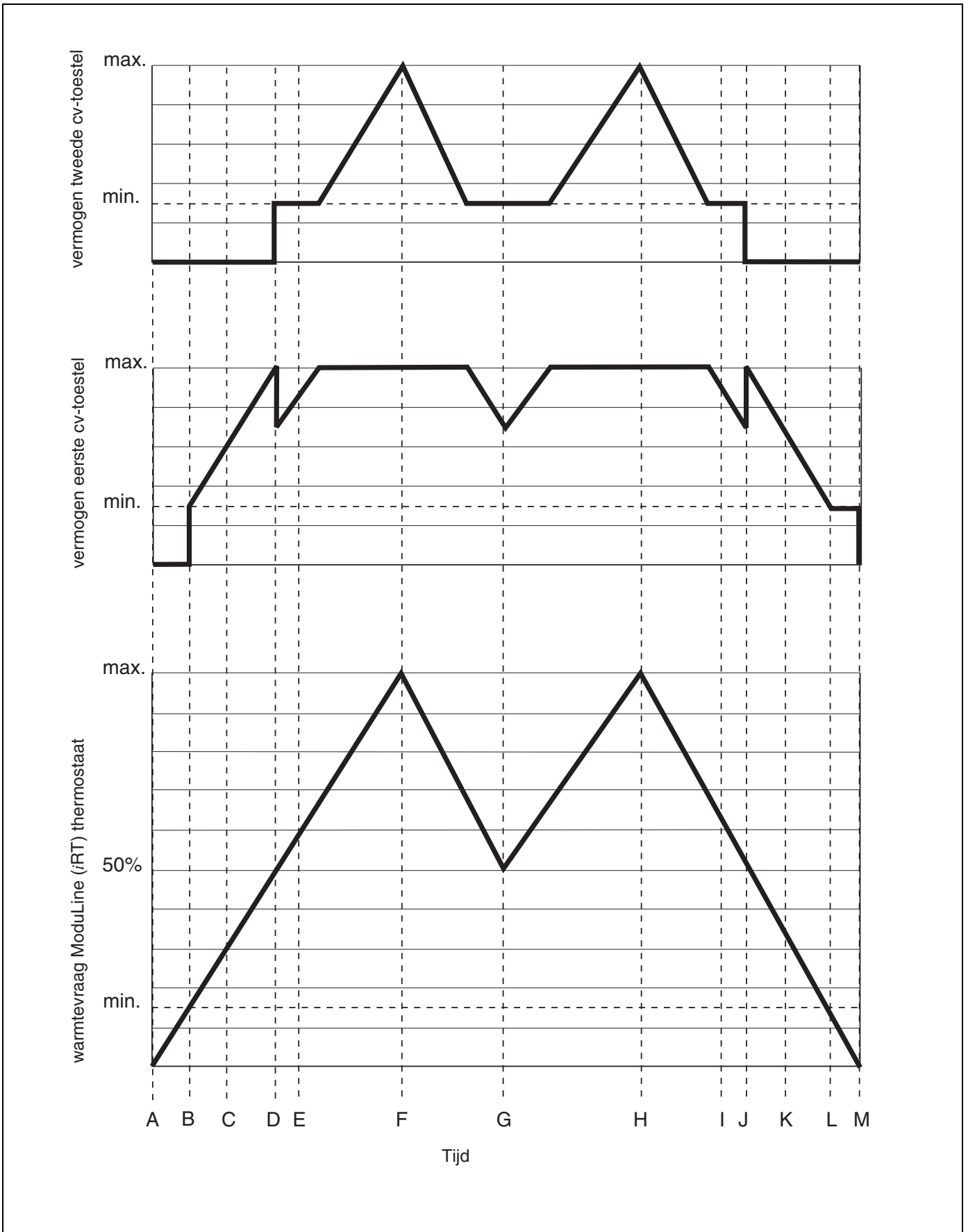
Fig. 4 Schakelmethode van de MBC 2 in combinatie met een modulerende weersafhankelijke regeling
