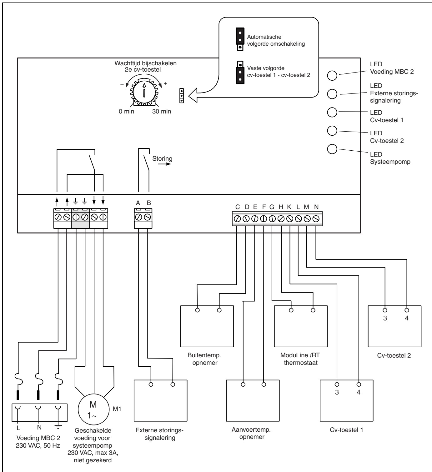
Fig. 8 Elektrische aansluiting en instellingen
