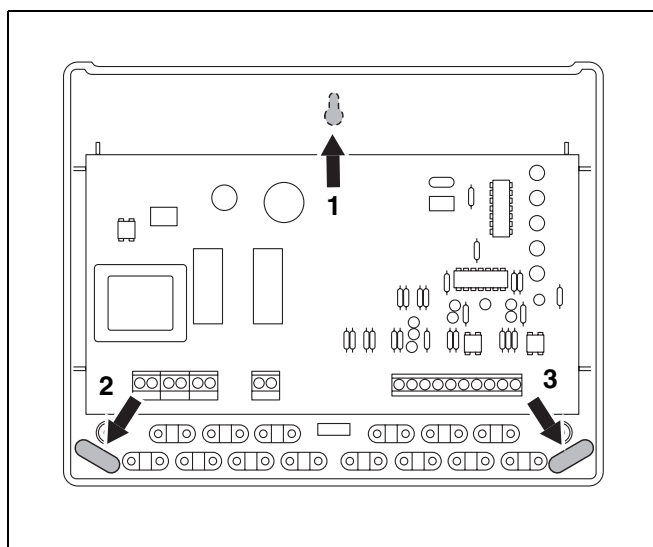
Fig. 7 Bevestigen van de MBC 2
