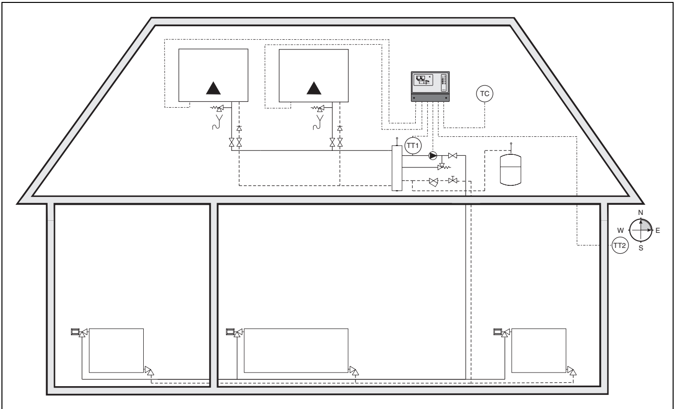
Fig. 3 Modulerende weersafhankelijke regeling
