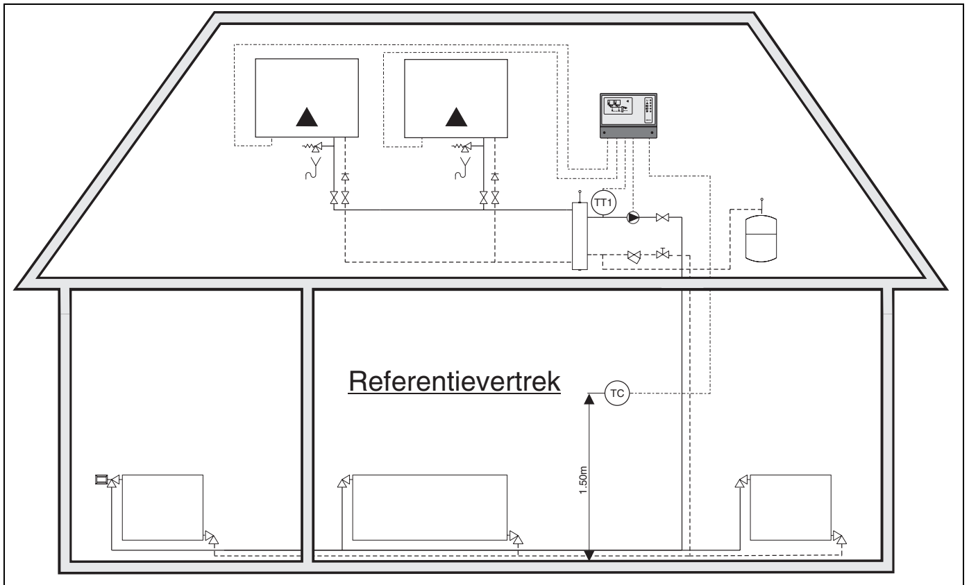
Fig. 2 Modulerende ruimtetemperatuurregeling
