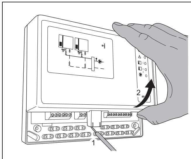
Fig. 6 Verwijderen bovenste afdekkap
