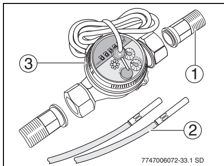
Afb. 6 Warmtehoeveelheidsteller
