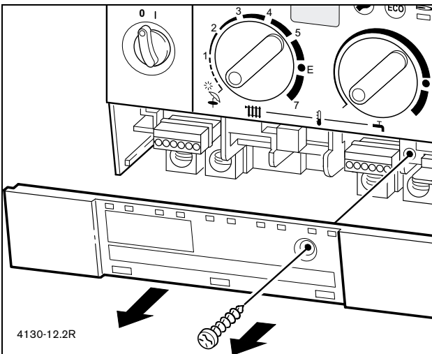
Afb. 6 Afscherming verwijderen
