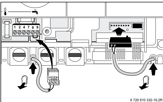
Afb. 7 Stekker van NTC 1 (links) en NTC 2 (rechts) vaststeken
