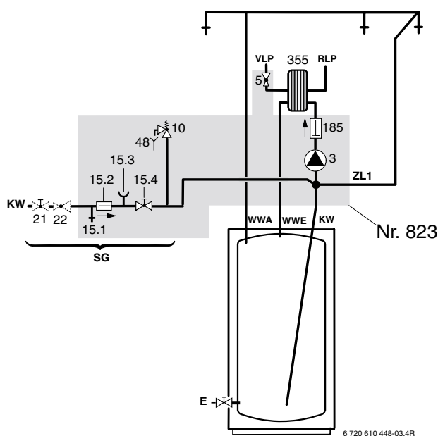
Afn. 3 Aansluitschema met circulatie ZL1
