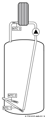
Afb. 1 Schema met NTC-posities
